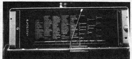
Unten: Die Skala des Geräts, auf der die Mittel- und Langwellenfelder nicht durcheinander, sondern übersichtlich nebeneinander stehen: Die fünf linken Spalten sind Mittelwellen-, die drei rechten Spalten Langwellen-Sender. Der Zeiger steht gerade in der Umschaltstellung.
