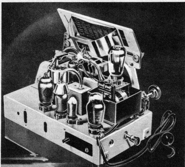
Der Innenaufbau des Vierröhren-Superhets ohne Wellenumschaltung. Sämtliche Photo: Werkphoto.
